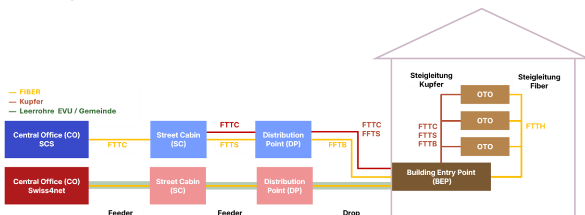
Abbildung 10: Central Office (CO) bis Anschluss Endkunden (OTO)
